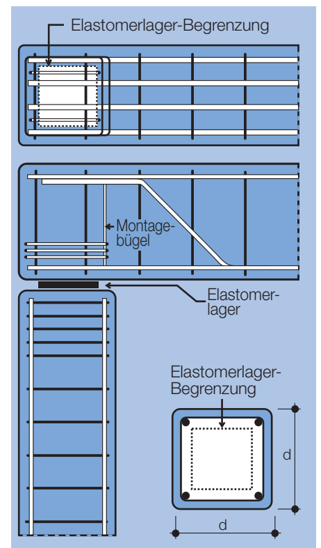
Bild 10: Methode B: Die Querkzugkräfte werden von einer den Bereich der Lagerfläche ringförmig umschließenden Bewehrung aufgenommen
