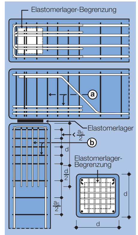
Bild 9: Methode A: Die Querkzugkräfte werden unmittelbar an ihrem Entstehungsort durch Bewehrung gedeckt. a) Binder-Querzugbewehrung: horizontale Schlaufen und Zusatzverbügelung b) Stützen-Querzugbewehrung: vertikale Schlaufen und Zusatzverbügelung, kreuzweise angeordnet
